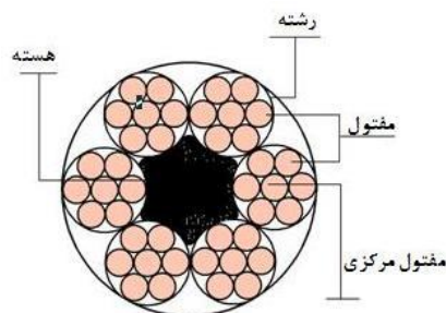
سطح مقطع سیم بکسل و اجزاء آن
